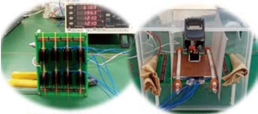
自然空冷測定
